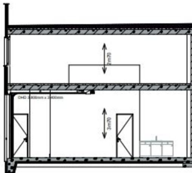
PRINCIPE DOORSNEDE
